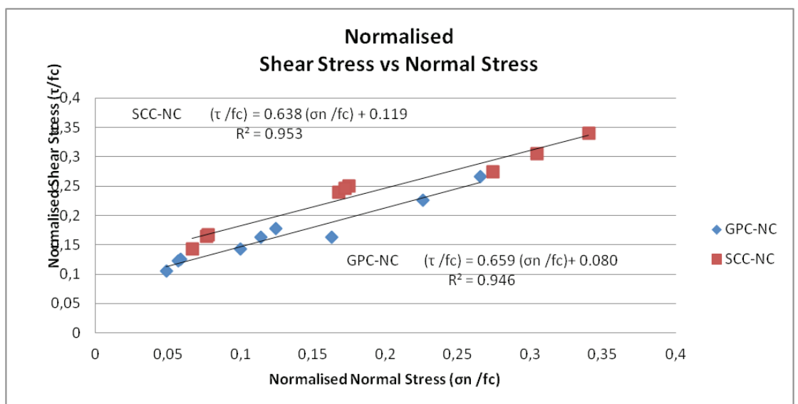
Rys. 7. Porównanie znormalizowanej zależności pomiędzy naprężeniem ścinającym i naprężeniem normalnym dla obu zestawów GPC-NC i SCC-NC
